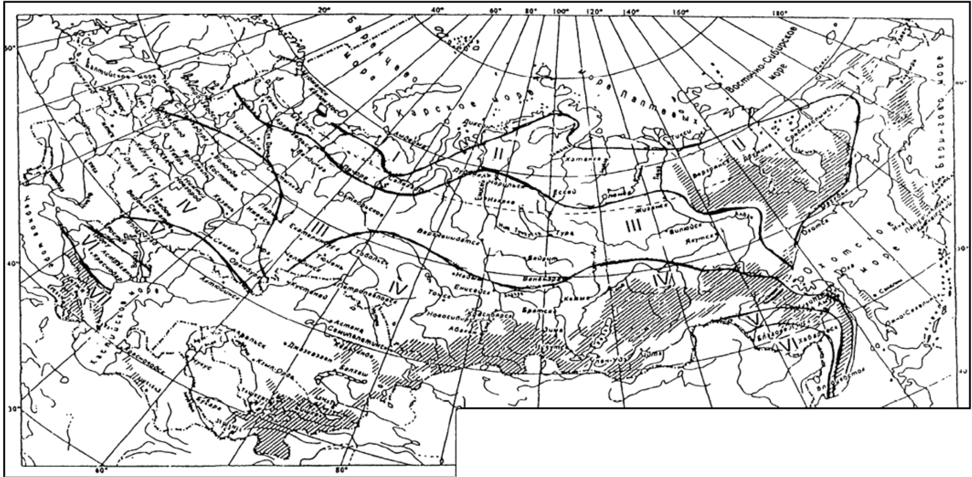
Рисунок А.5 - Схематическая карта районирования по величине удельной энтальпии h , кДж/кг, наружного воздуха в теплый период года (параметры Б): I - h \leq 44 ; II - h = 44 - 48,4 ; III - h = 48,4 - 52,6 ; IV - h = 52,6 - 56,8 ; V - h = 56,8 - 61 ; VI - h = 61 - 65 ; VII - h = 65 - 69
